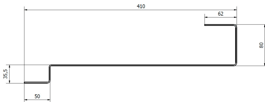
RYS.1 RZUT Z BOKU
