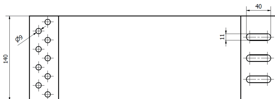
RYS.2 RZUT Z GÓRY
