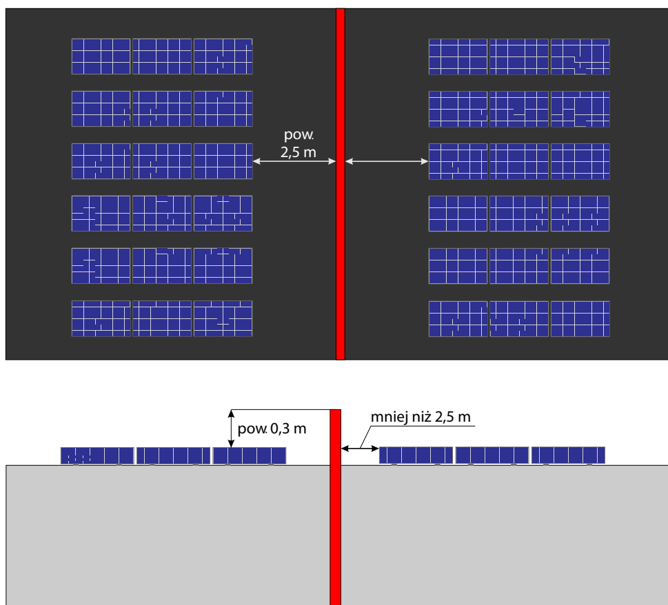
RYS. 3. Usytuowanie modułów PV względem ściany oddzielenia przeciwpożarowego.
